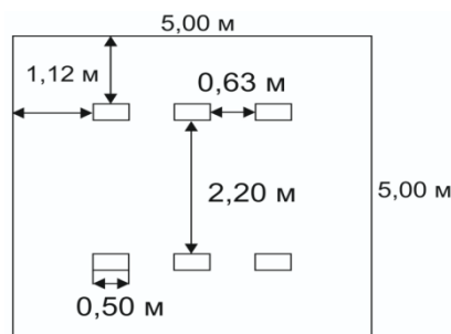
Рисунок 5.2 – План помещения и размещения светильников с люминесцентными лампами
