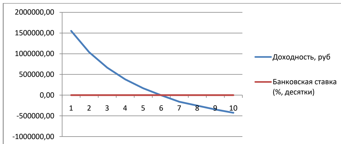
Рисунок 4.4 Зависимость NPV от ставки дисконтирования
